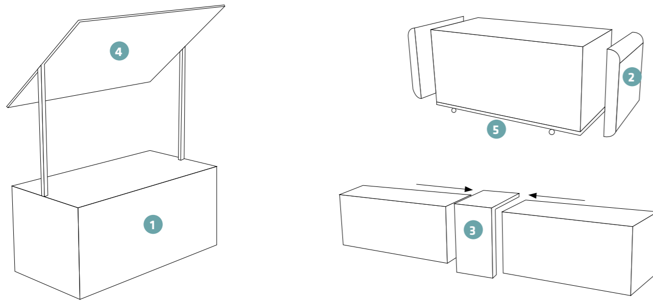
1 Buffet 2 Joues 3 Raccord 4 Toit 5 Socle à roulettes
